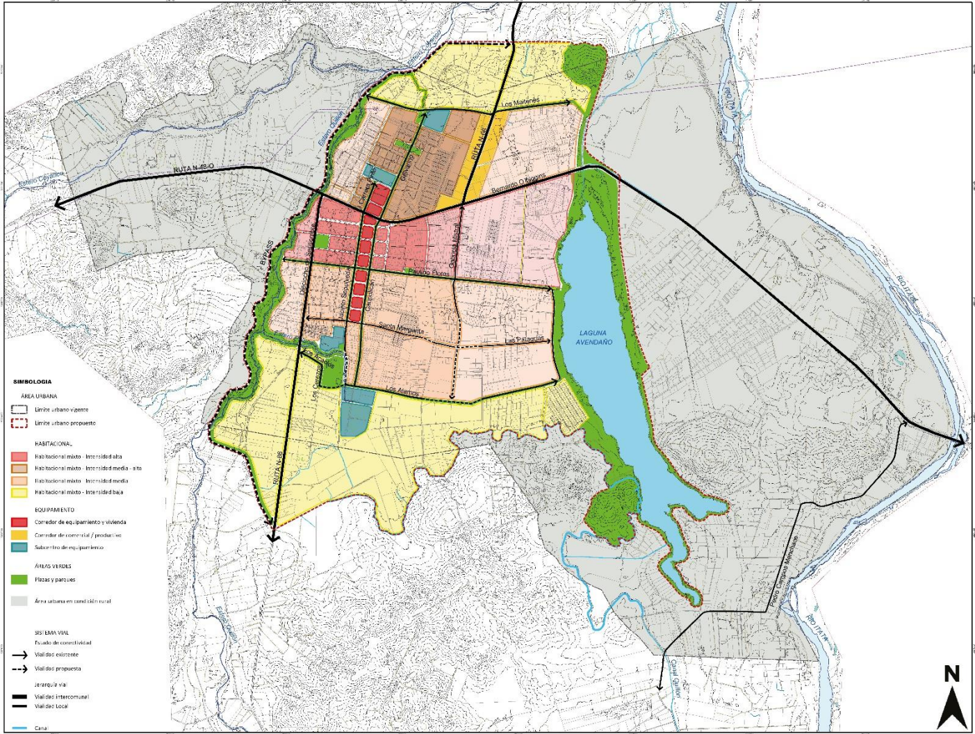
Figura 61: Alternativa 1 - Ejes Conectores Norte - Sur
