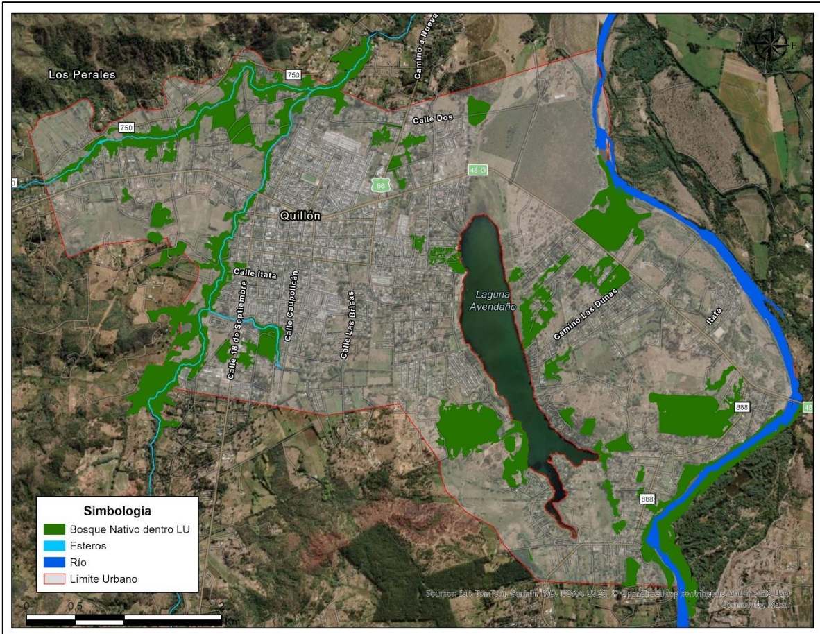
Figura 12: Localización y Distribución del Bosque Nativo dentro del Límite Urbano en Quillón
