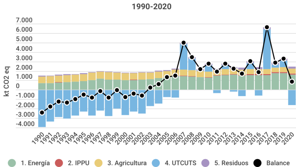
Figura 18: Emisiones y absorciones de GEI (kt Co2eq) de alcance 1 por sector, 1990 - 2020
