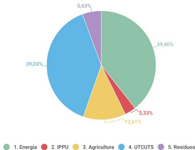
Figura 19: Emisiones y absorciones de GEI (kt Co2eq) de alcance 1 por sector, 2020
