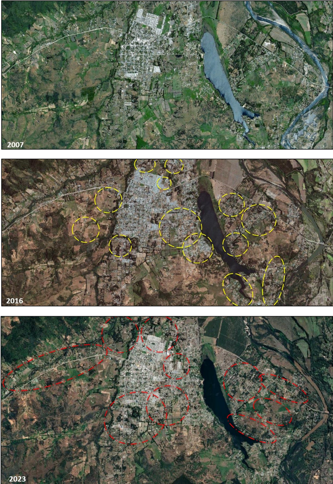
Figura 37: Ocupación territorial entorno a áreas urbanas consolidadas, cuerpos de aguas y vías de conectividad años 2007, 2016 y 2023, comuna de Quillón.
