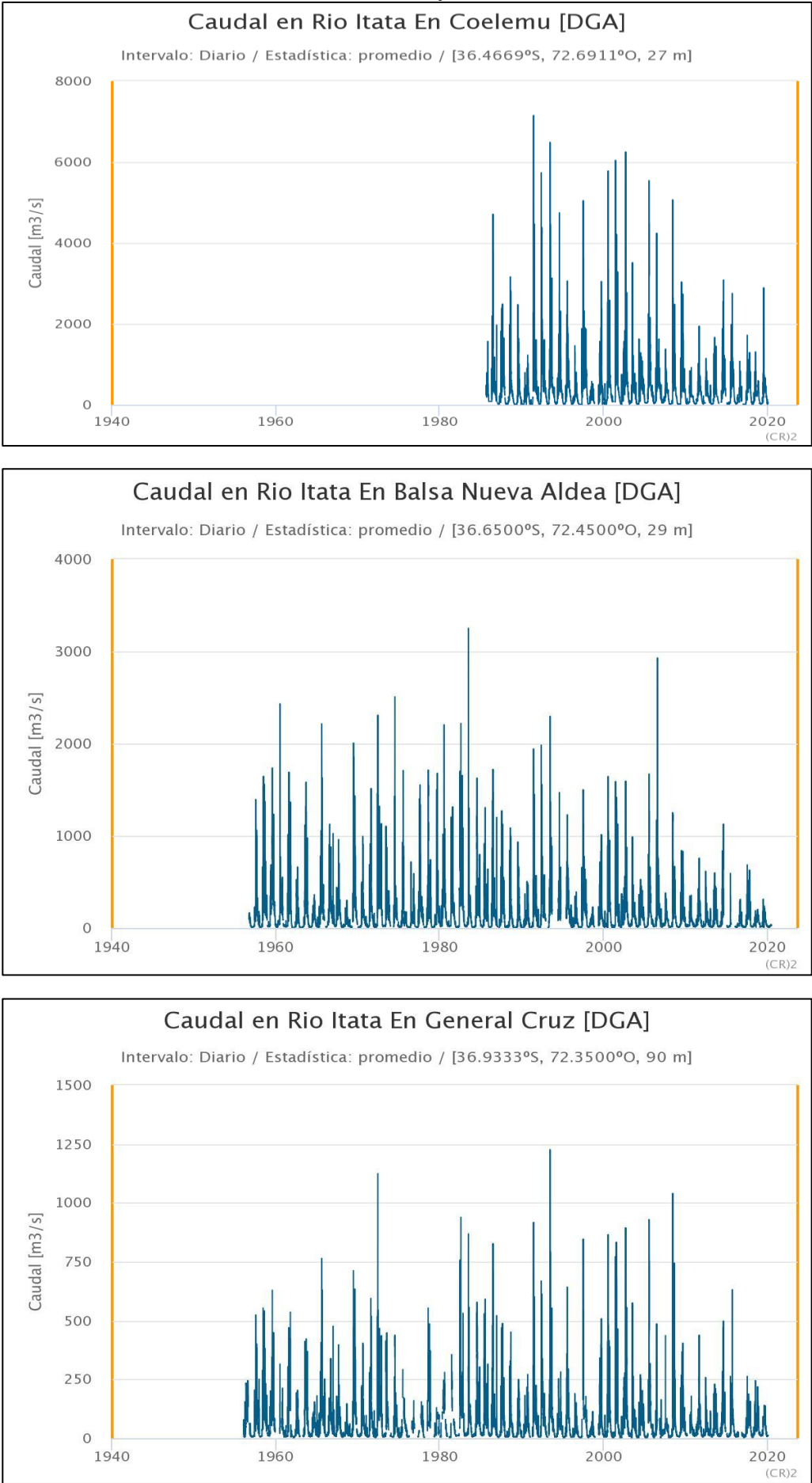
Figura 51 : Caudales del Río Itata de las estaciones fluviométrica de Coelemu, Nueva Aldea y General Cruz, entre los años 1956 y 2020.
