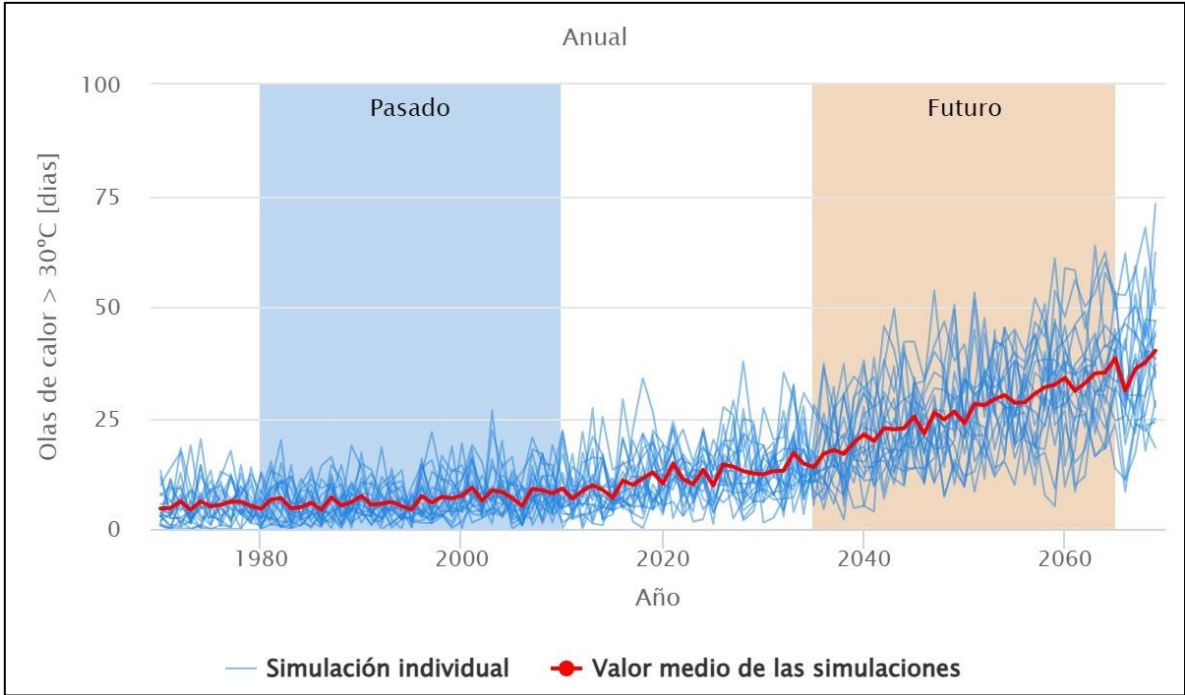
Figura 49: Variación en las Olas de Calor en Quillón
