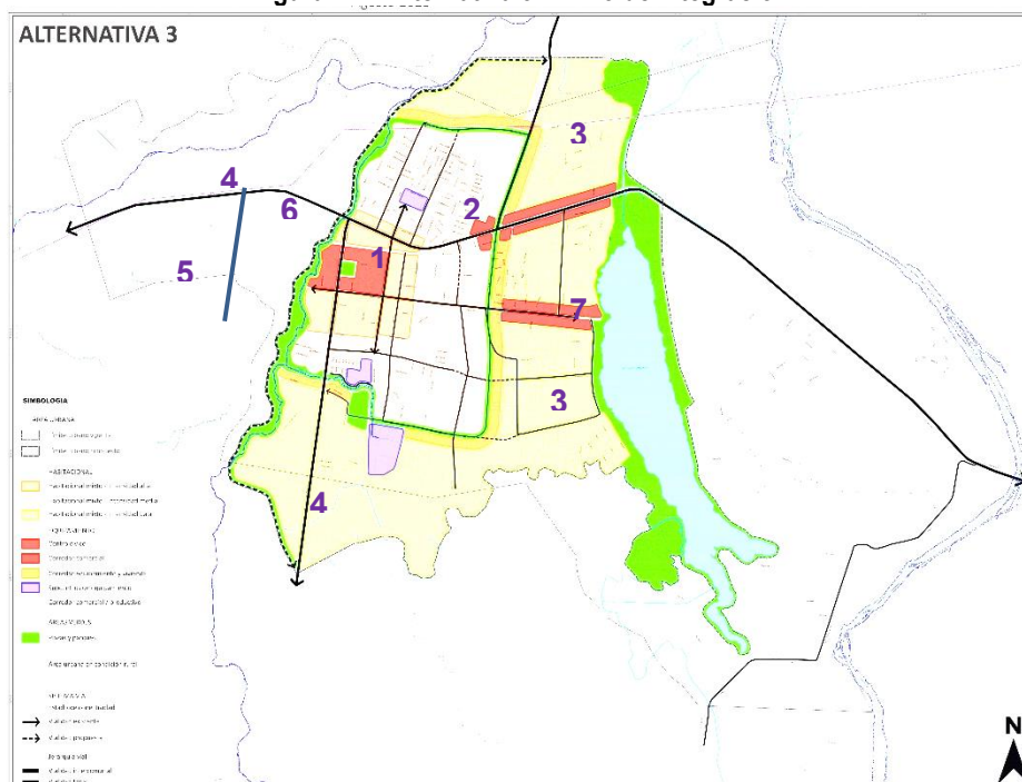
Figura 117: Alternativa 3: Anillo de integración
