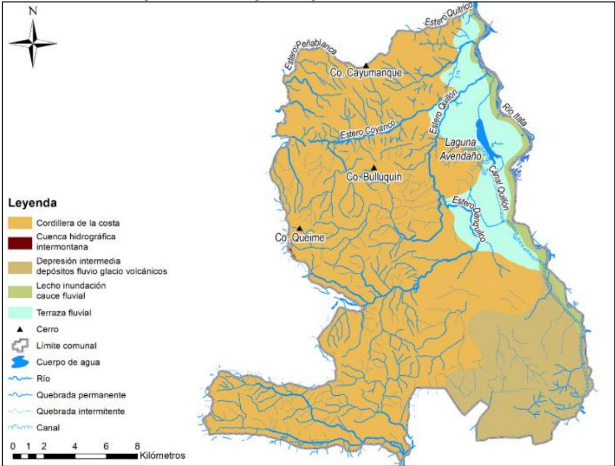
Figura 10: Geomorfología e hidrografía de la comuna de Quillón
